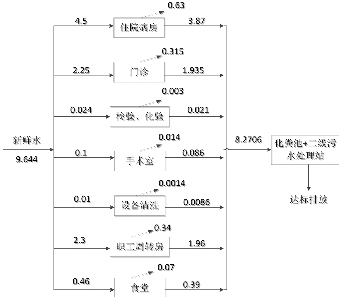
图3-5 运营期水量平衡图
